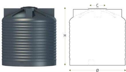
RESERVATÓRIOS SUBTERRÂNEOS VERTICAIS (RSV)
