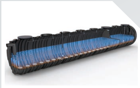
STATION D'EPURATION MONOBLOC A BOUES ACTIVEES (50 A 10.000 EH)
