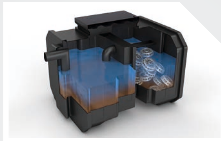
FILIERE FILTRE COMPACT MONOBLOQUE
