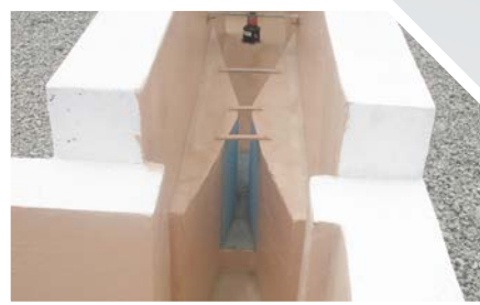
DEBITMETRES A ULTRASON ET CANAL VENTURI | CANAL PARSHALL PRÉFABRIQUE
