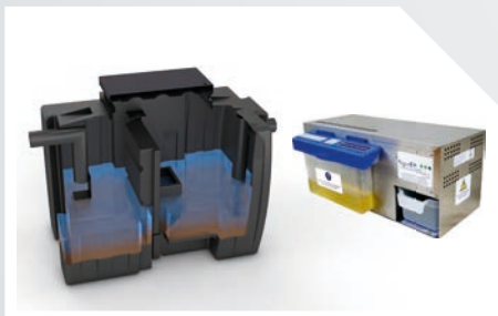
SEPARATEURS DE GRAISSES
