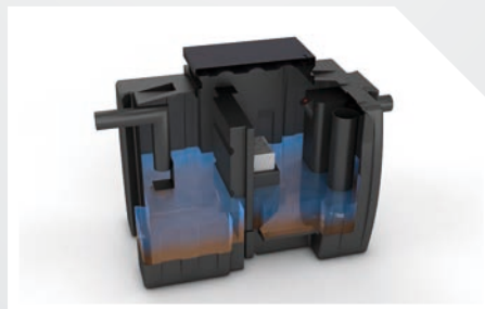
SEPARATEURS D'HYDROCARBURES
